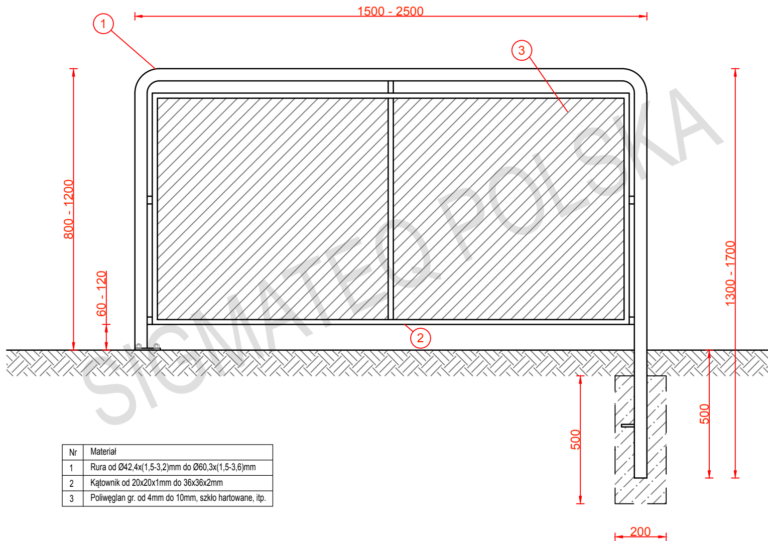
Rysunek nr 12 – Bariery z rur przeciwbryzgowie / przeciwbłotne
