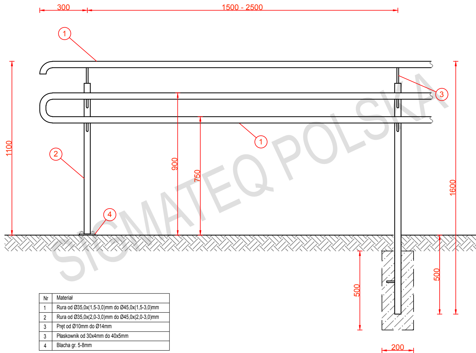
Rysunek nr 9 – Balustrady i poręcze z pochwytyami dla niepełnosprawnych
