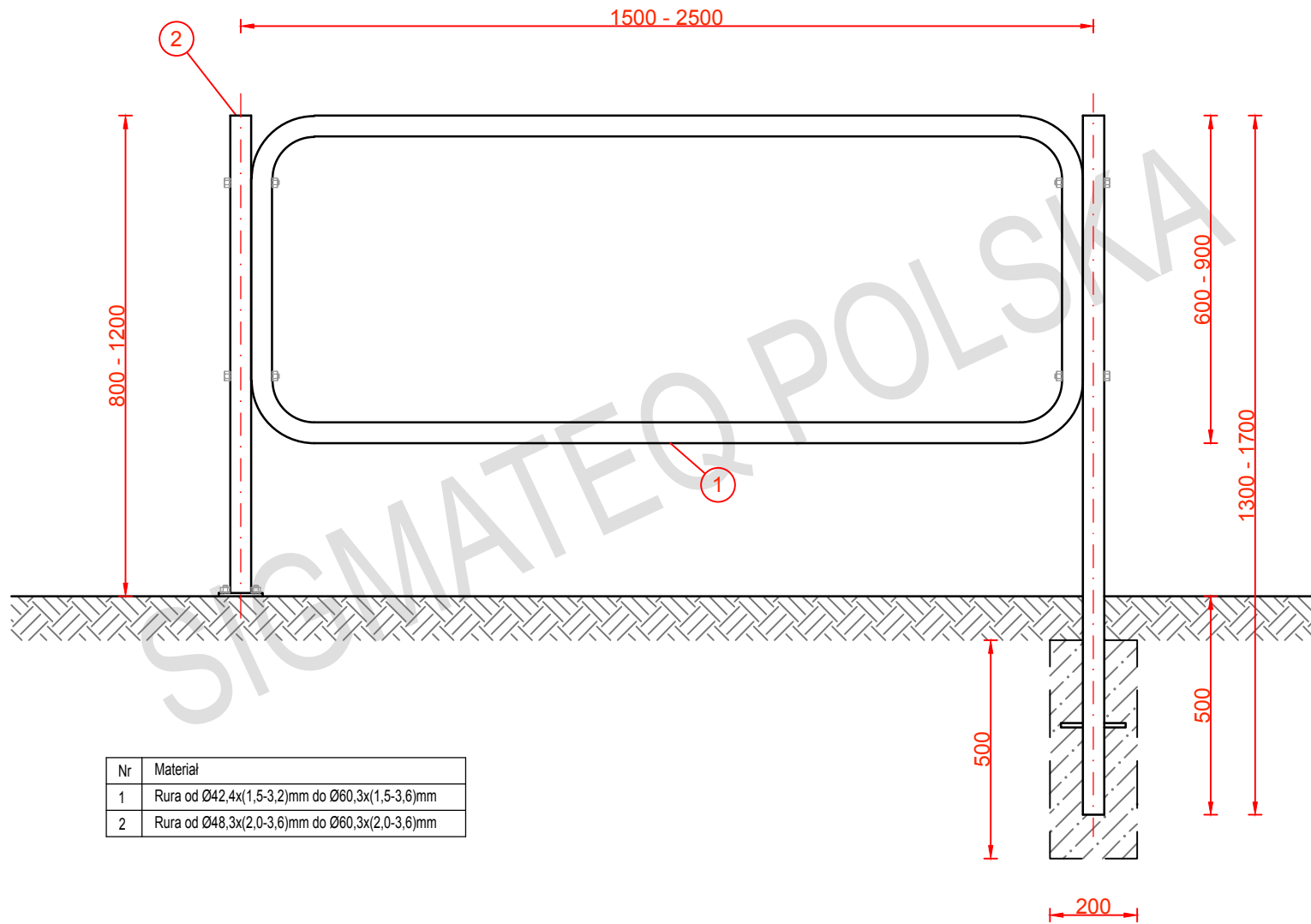
Rysunek nr 8 – Bariery z rur na słupkach typu "0"
