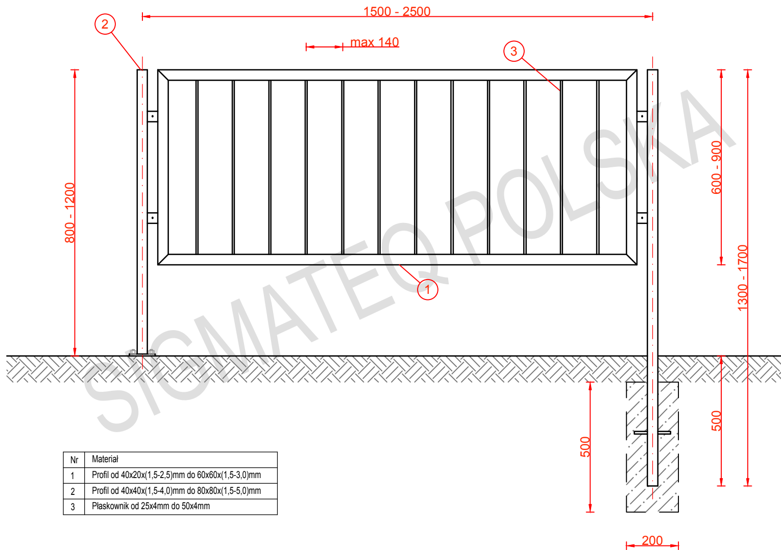
Rysunek nr 6 – Bariery z kątowników i płaskowników
