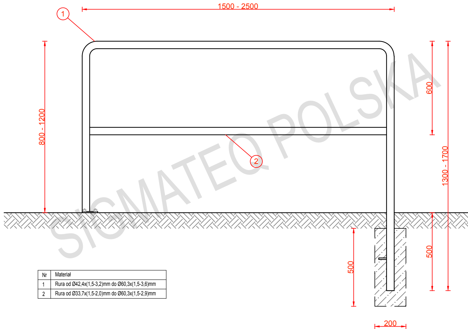
Rysunek nr 5 – Bariery z rur z poziomym przeciągiem
