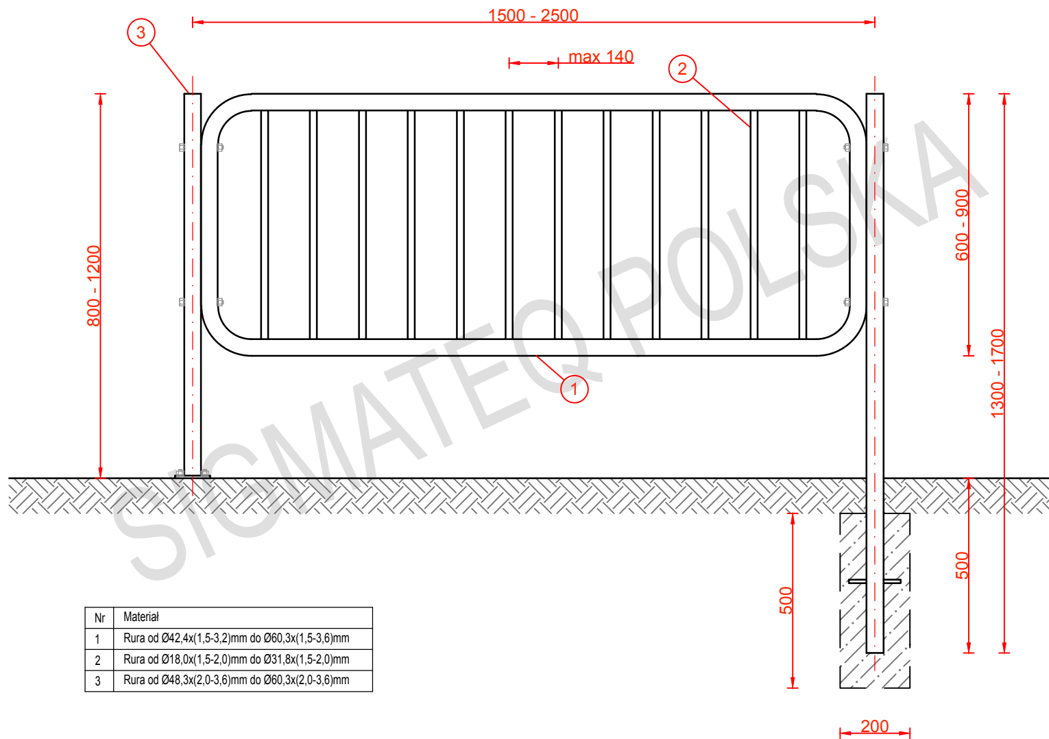
Rysunek nr 4 – Bariery z rur na słupkach
