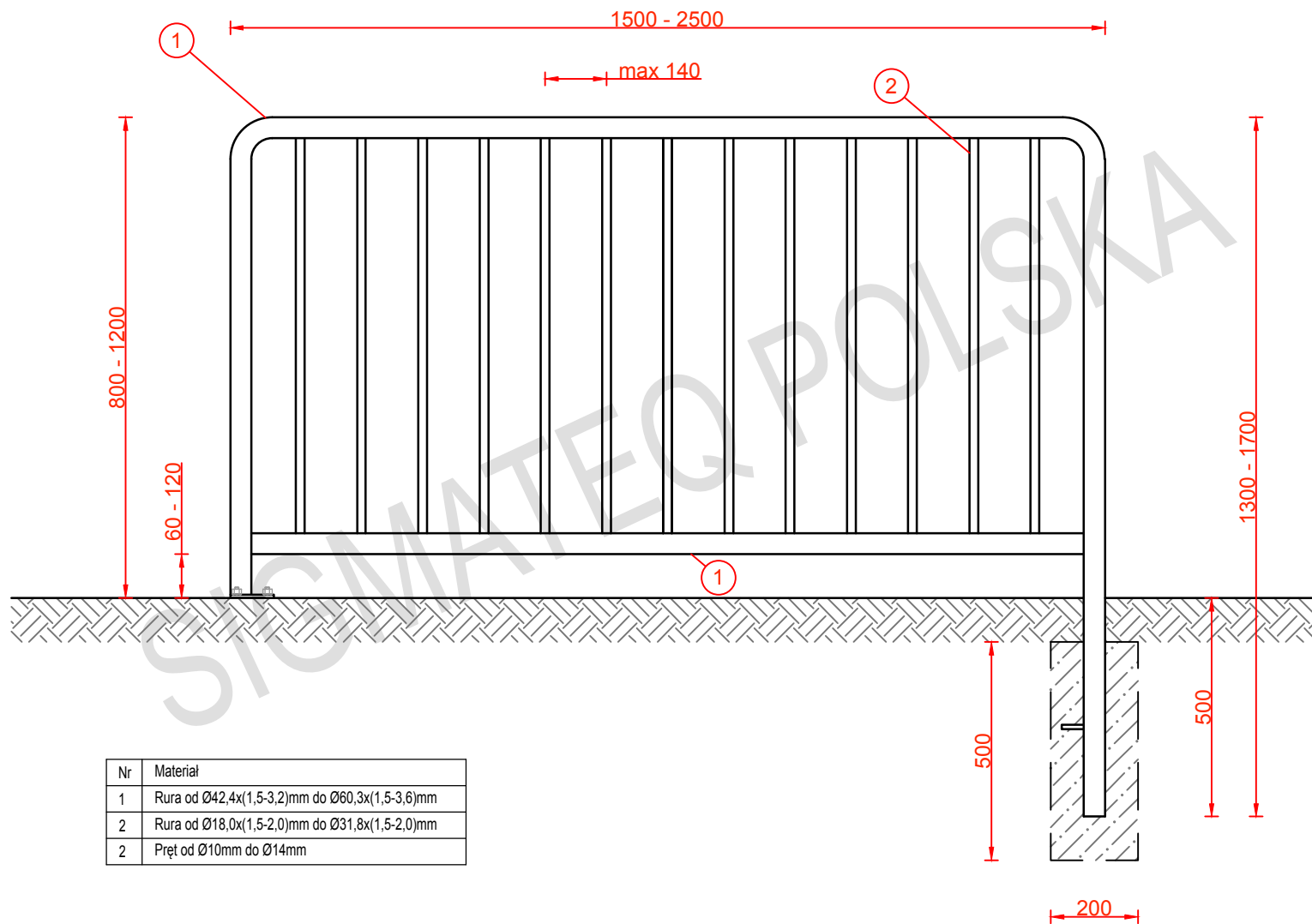
Rysunek nr 3 – Bariery z rur
