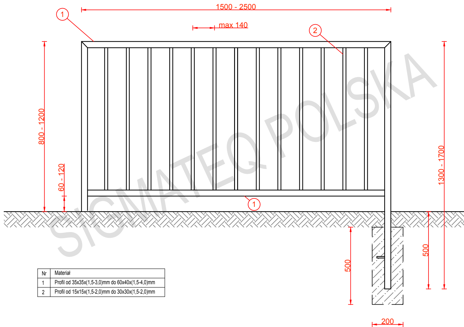
Rysunek nr 2 – Bariery z kątowników
