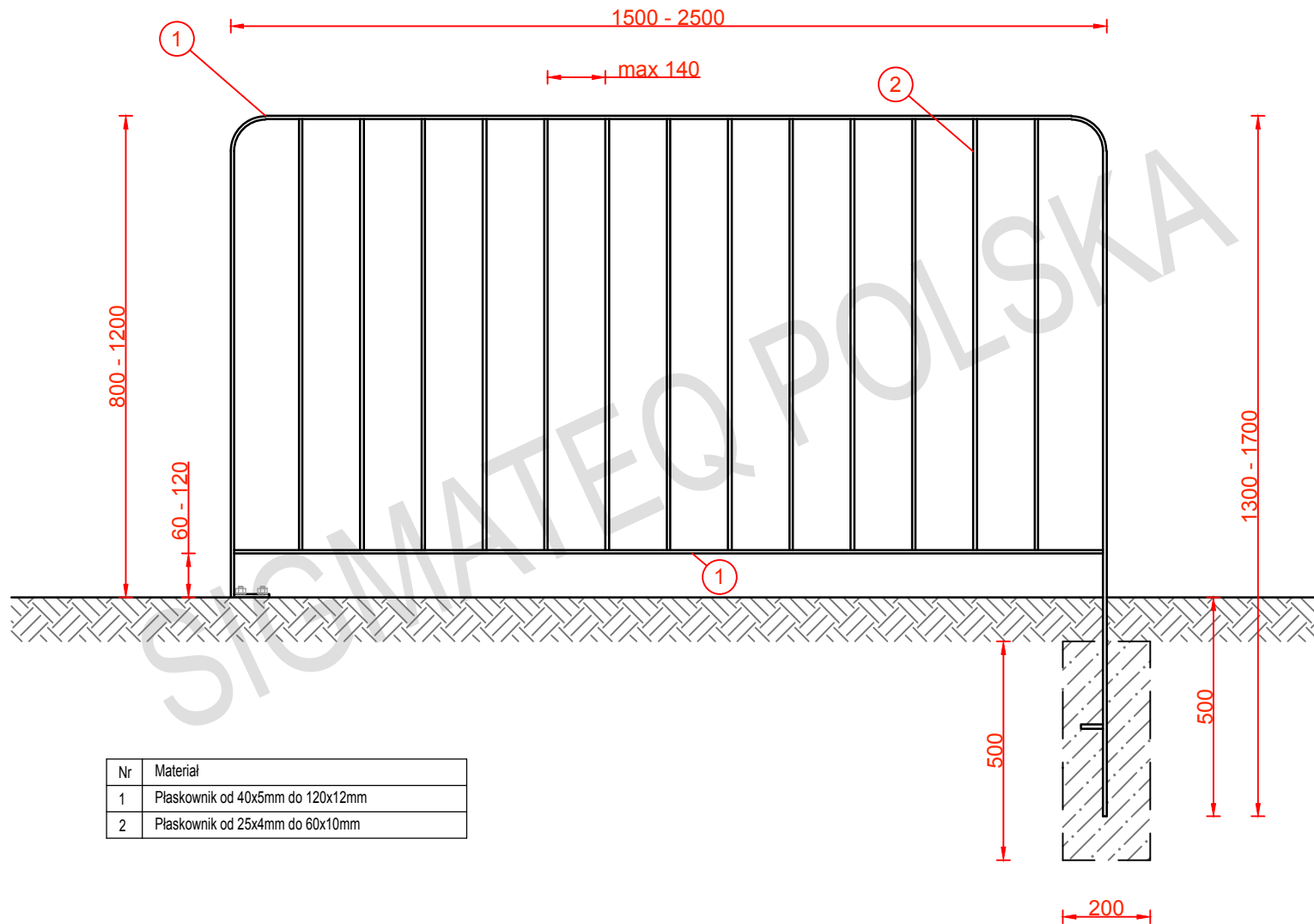
Rysunek nr 1 – Balustrady z płaskowników
